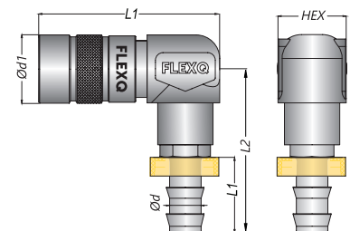
Kupplung mit 90° Schnellsteck - Schlauchtülle
