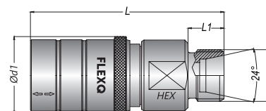
Cone 24°
