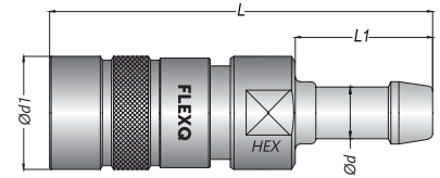
Kupplung mit gerader Standard - Schlauchtülle
