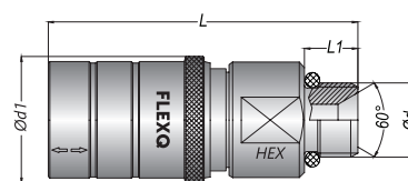
60° Konus
