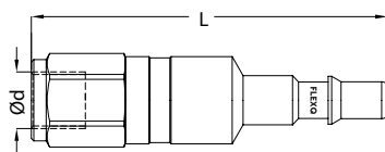
Verschlussnippel mit Innengewinde
