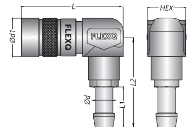
Kupplung mit 90° Standard - Schlauchtülle
