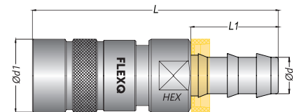
Kupplung mit gerader Schnellsteck - Schlauchtülle
