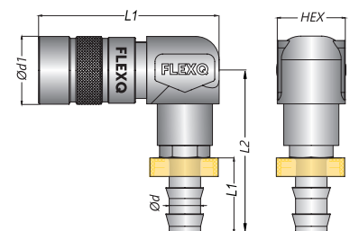
Kupplung mit 90° Schnellsteck - Schlauchtülle
