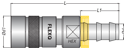
Push to connect hose tail socket / Kupplung mit gerader Schnellsteck - Schlauchtülle
