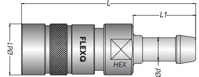
Standard hose tail socket / Kupplung mit gerader Standard - Schlauchtülle
