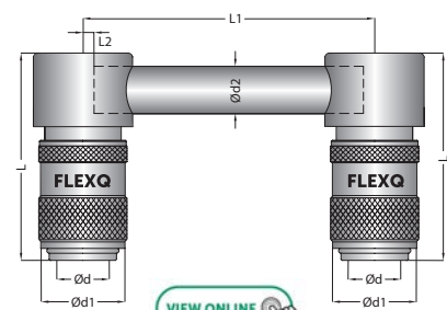
Diverting sockets / Umlenkkipplung
