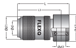
Diverting sockets / Umlenkkipplung
