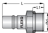
Short version for screwing into the multi-coupling blocks Kurze Version zum Einschrauben in die Multikupplungsblöcke
