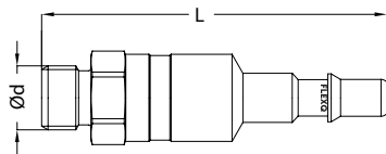
Verschlussnippel mit Außengewinde
